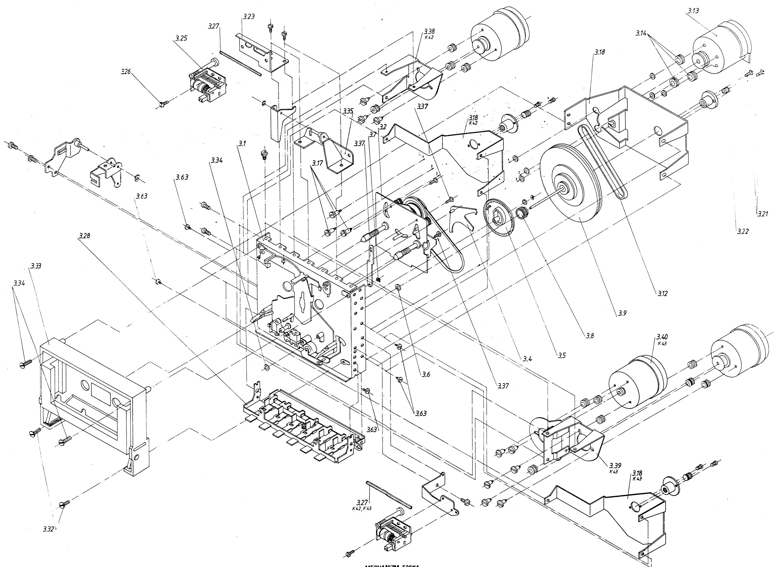
МЕХАНИЗМ 520K4
